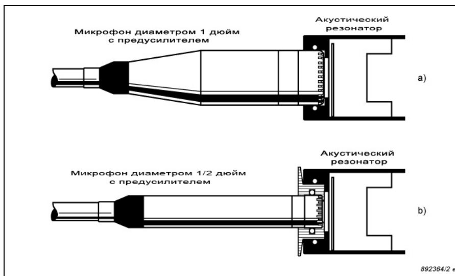
Рис. 2. Подключение микрофонов компании В&К к акустическому резонатору.
